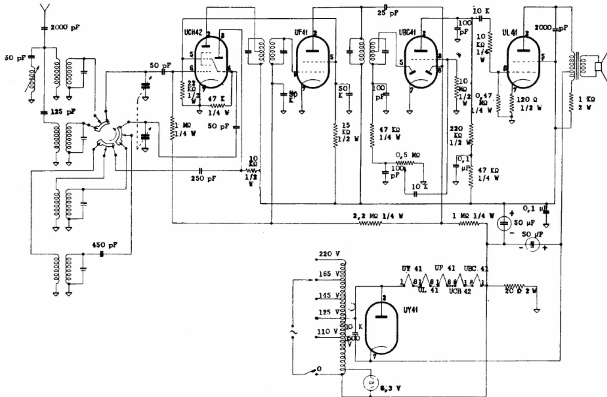
IRRADIO - Mod. EN 40. Onde medie e cort. Media frequenza a 467 kc/s. Potenza indistorta di uscita 2 watt. Consumo 32 watt.
